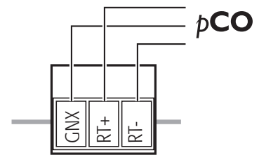
PHOENIX® MC1,5/3-ST-3,81
