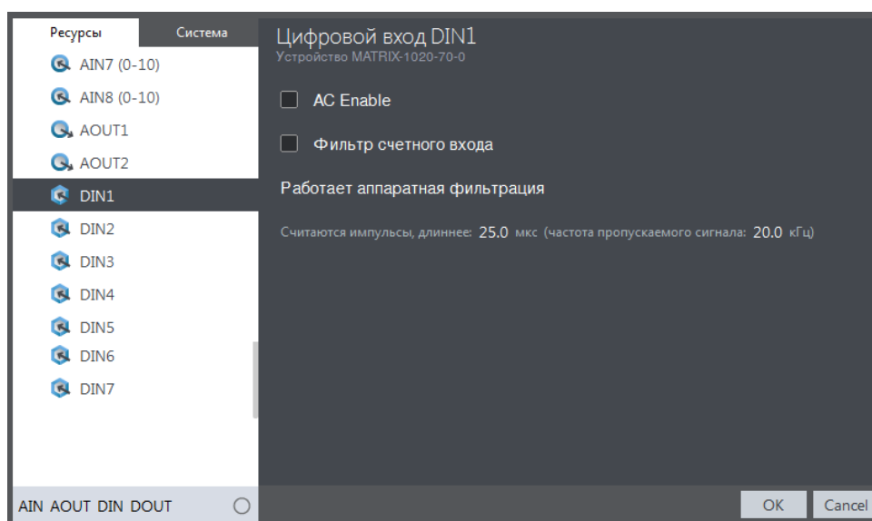
Рис. 62 - Конфигурирование DIN
