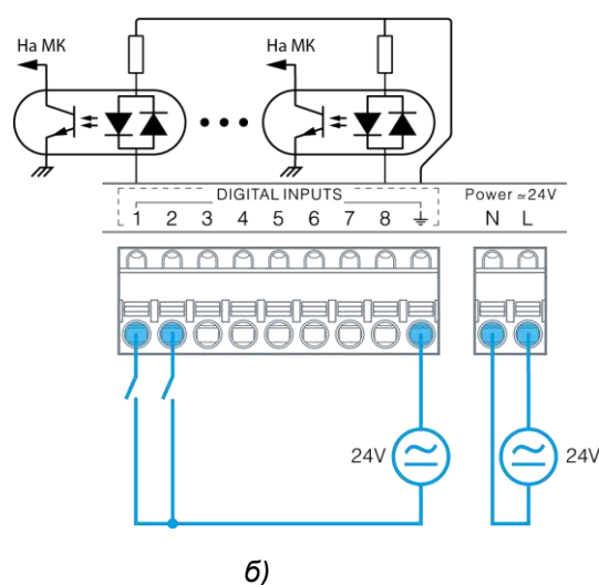
Рис. 9 – Питание дискретных датчиков и контроллера от одного источника (а); от отдельных источников (б)
