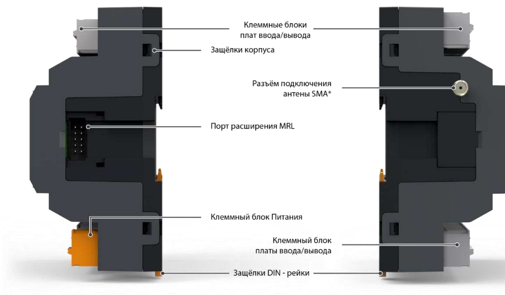
Рис. 3 –Контроллер Matrix. Виды сбоку
