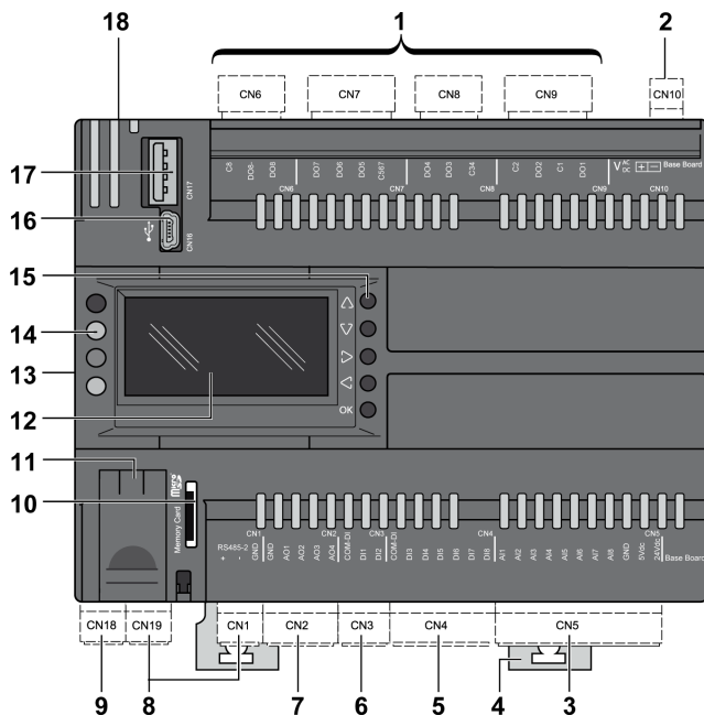
Контроллер TM172P•28•:
