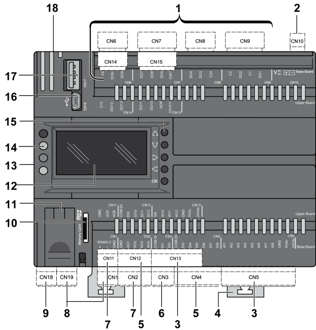
Контроллер TM172P••42••:
