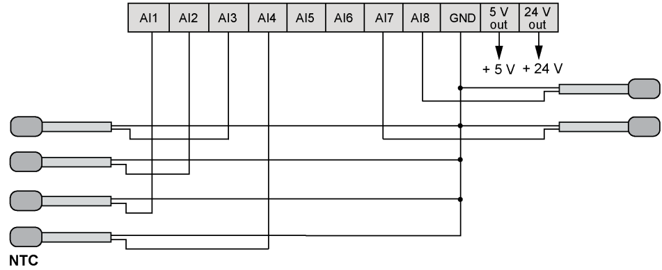
Подключение входа NTC TM172•••28•• / TM172•••42•• CN5:
